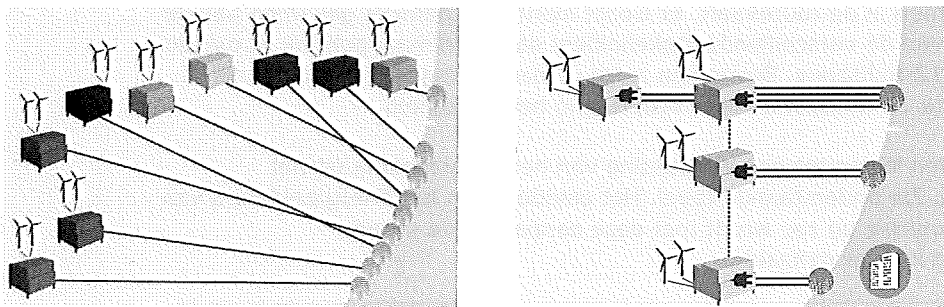
Schematische weergave van individuele aansluiting (links) en een net op zee (rechts).
